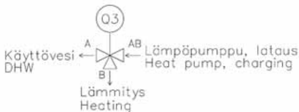
Vaihtventtiili/zone valve: VRBI60.xx Toimilaite/actuator: GMA321
