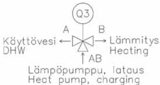
Vaihtventtiili/zone valve: LK525 Toimilaite/actuator: EMV 110-M
