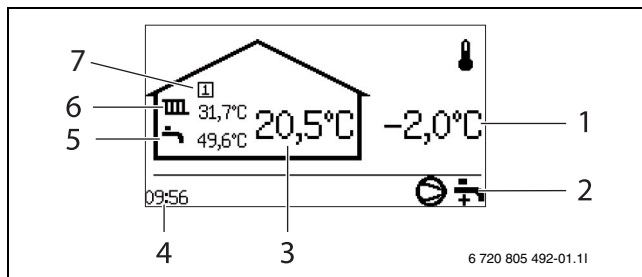
Kuva 3 Lähtötila
